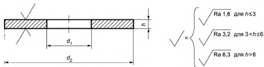
Рисунок 1 — Размеры
